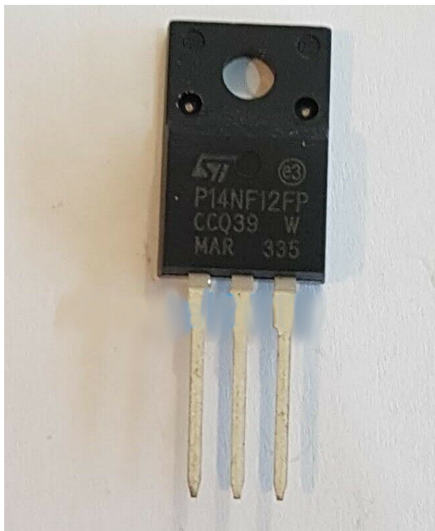
Transistor Mosfet N STP14NF12FP 120V 14A TO220F
