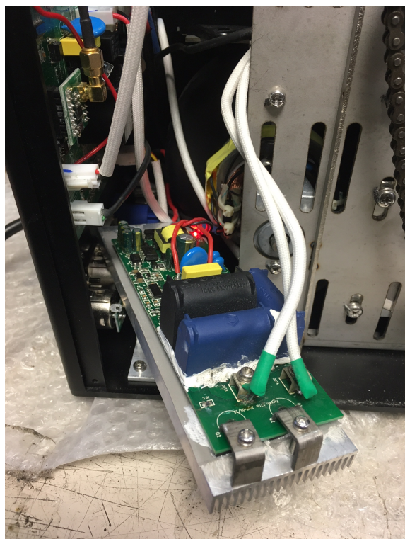
Carte PCB heater pour machine à étincelles Sparkle V2
