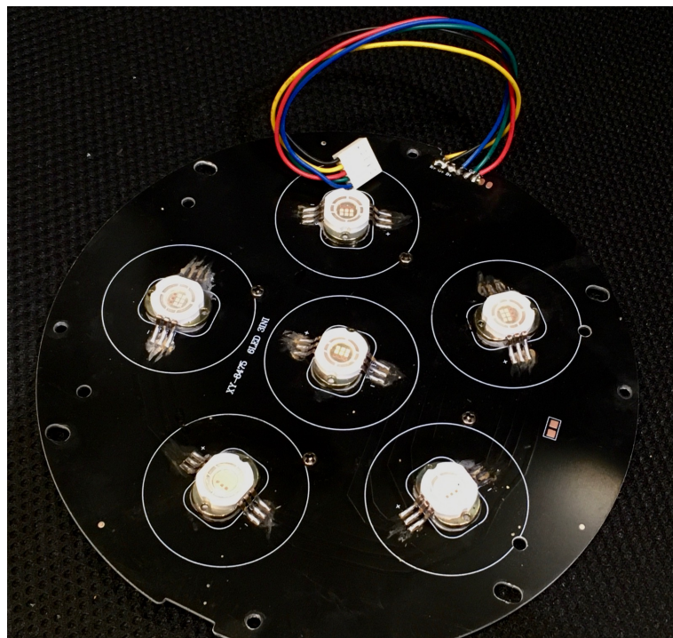
Carte Led pour COB630 Nicols
