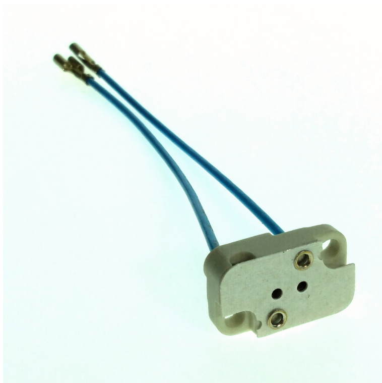
Douille GX5.3 Pro 13cm de fil avec cosses
