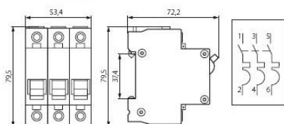
Disjoncteur triphasé 32A courbe B
