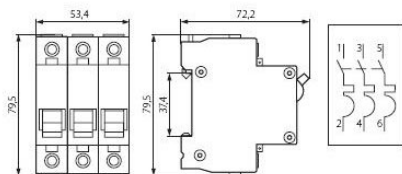
Disjoncteur triphasé 16A courbe B
